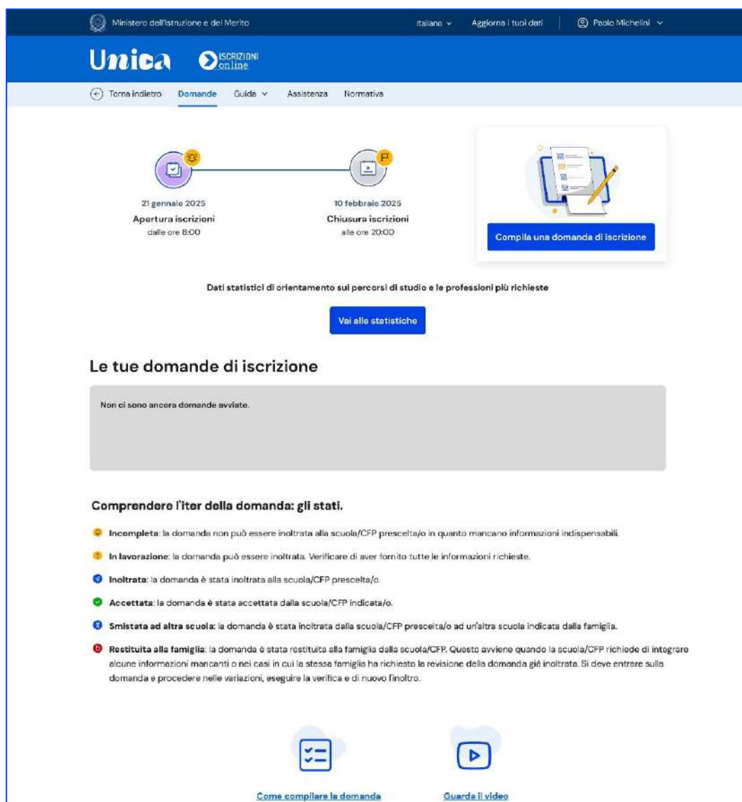
FIGURA 11 – SCHERMATA DOMANDE
